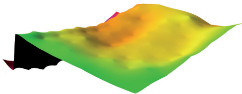
Abb. 1: Das Erdmagnetfeld in 3D unter denselben Einflüssen mit NIPNetz von TOP-QUANT.
